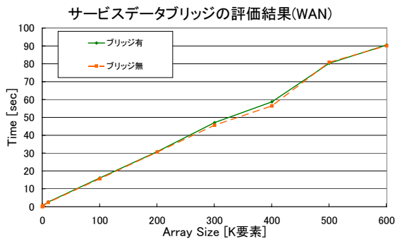
図 14 サービスデータブリッジの評価結果
