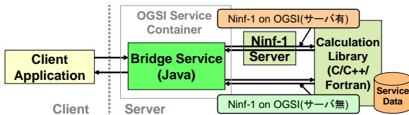
図 6 Ninf-1 on OSGI システム図
