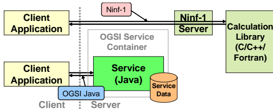
図 7 OSGI の Java 環境と Ninf-1 による RPC システム
