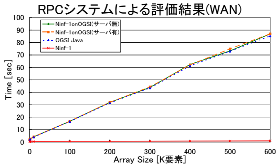
図 13 RPC システムによる評価結果
