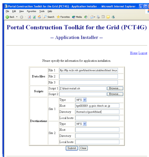
図 2 アプリケーションインストール画面
