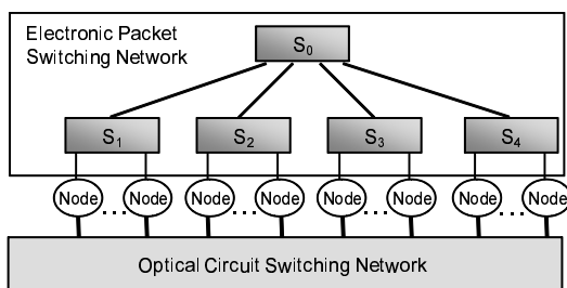
図 1: 光・電気ハイブリッドネットワーク
